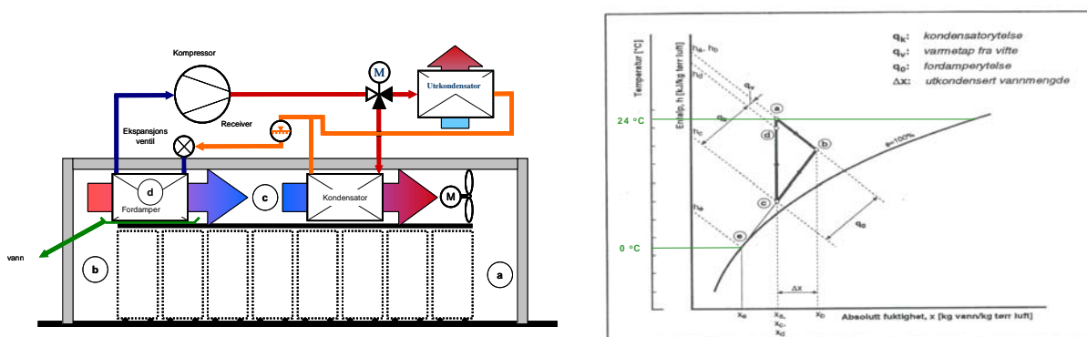
Figur 3: Prinsipp for varmepumpe ved klippfisktøking. A: Langblåst tørke. B: Tørkeprosessen i energi – vann diagrammet for fuktig luft.
